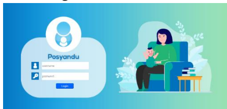
Gambar 3. Login
