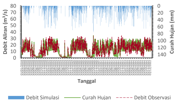
Gambar 4. Hidrograf Debit Simulasi Dan Observasi Hasil Validasi Sumber : Pengolahan hasil analisis SWAT, 2023
