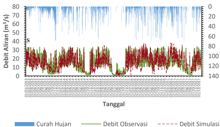
Gambar 2. Hidrograf debit simulasi dan observasi hasil kalibrasi Sumber : Pengolahan hasil analisis SWAT, 2023
