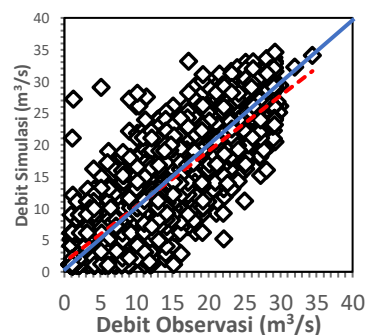
Gambar 5. Sebaran Debit Simulasi Dan Observasi Hasil Validasi Sumber : Pengolahan hasil analisis SWAT, 2023
